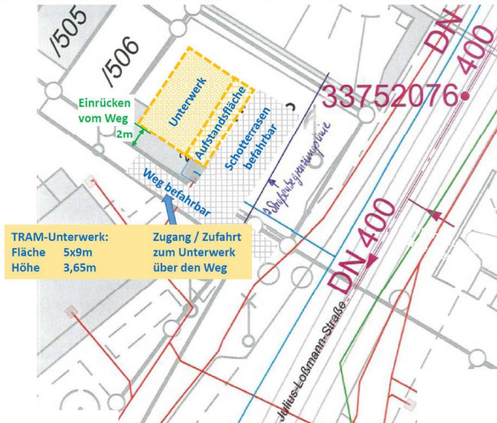
Abbildung 4 UW Finkenbrunn Lageplan
