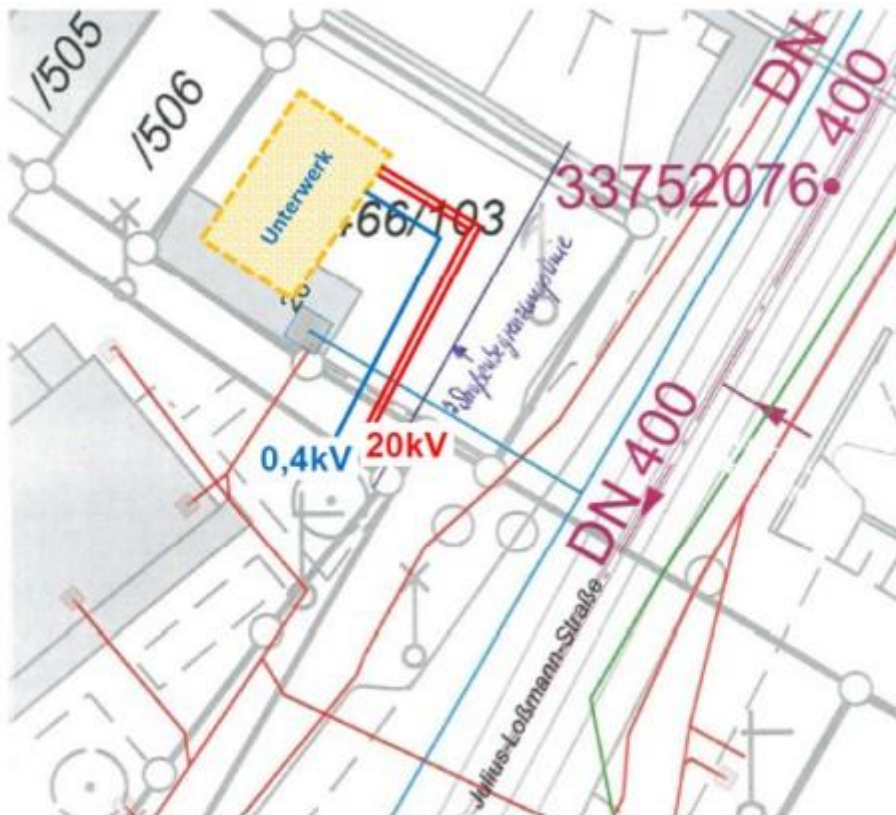
Abbildung 9 UW Finkenbrunn Einspeisung aus dem Netz des Energieversorgers
