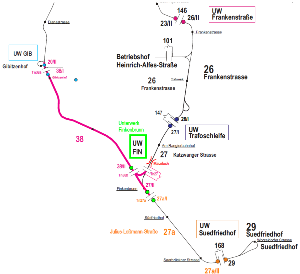
Abbildung 8 Auszug aus der Anlage 1.1 Minerva_F_Speisebezirksplan mit zusätzlichem UW Finkenbrunn
