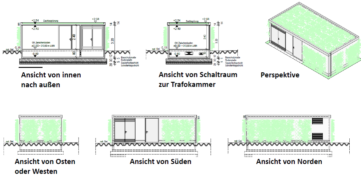
Abbildung 5 Finkenbrunn Gebäude und Ansichten
